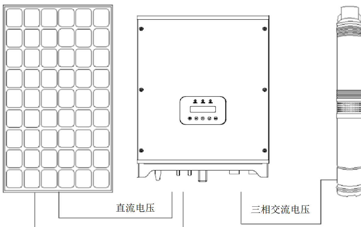
图 1-1 光伏扬水系统结构
