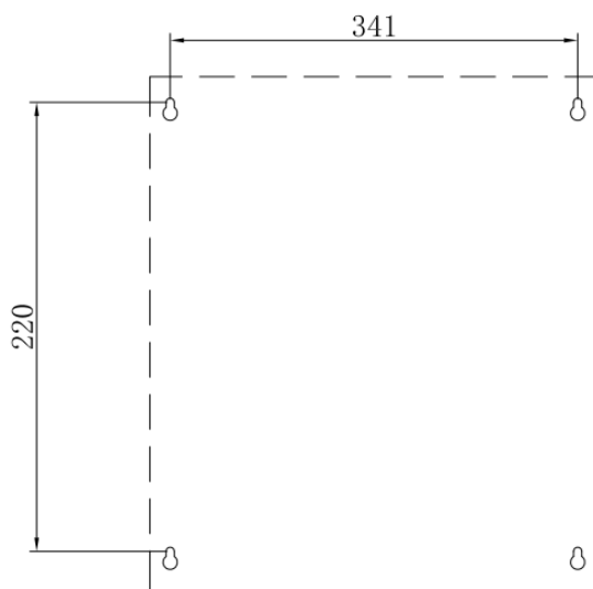
图 2-3 LWS 3000~5500 和 LWS 3000-A~5500-A 安装尺寸
