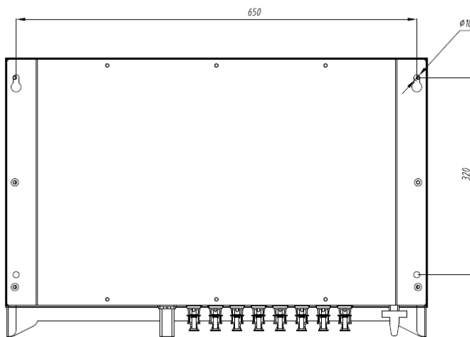
图 2-6 LWS 37K~55K 和 LWS 37K-A~55K-A 安装尺寸
