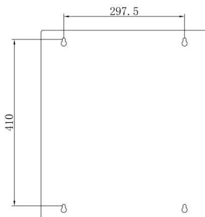
图 2-5 LWS 15K~30K 和 LWS 15K-A~30K-A 安装尺寸
