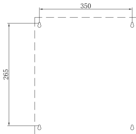
图 2-4 LWS 7500~11K 和 LWS 7500-A~11K-A 安装尺寸
