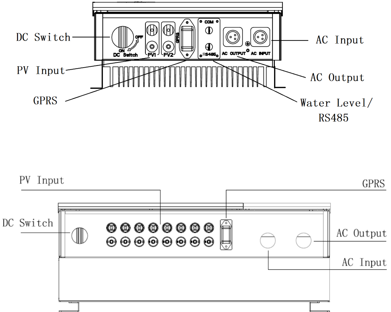
图 2-7 LWS 产品接线图
