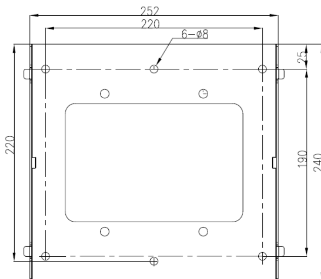
图 2-2 LWS 1500-L~2200-L 和 LWS 1500-LA~2200-LA 安装尺寸
